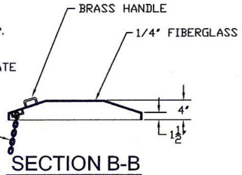
SNUFFER TRAY LID
