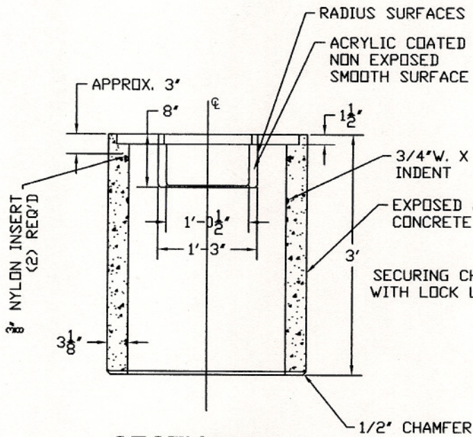
SECTION A-A RECEPTACLE
