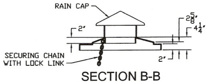
TRASH RECEPTACLE LID
